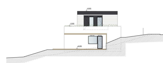
POHLED JIŽNÍ
